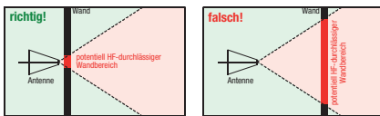
Abbildung: Illustrationsskizze zur Ortungsunsicherheit bei Messantennen
